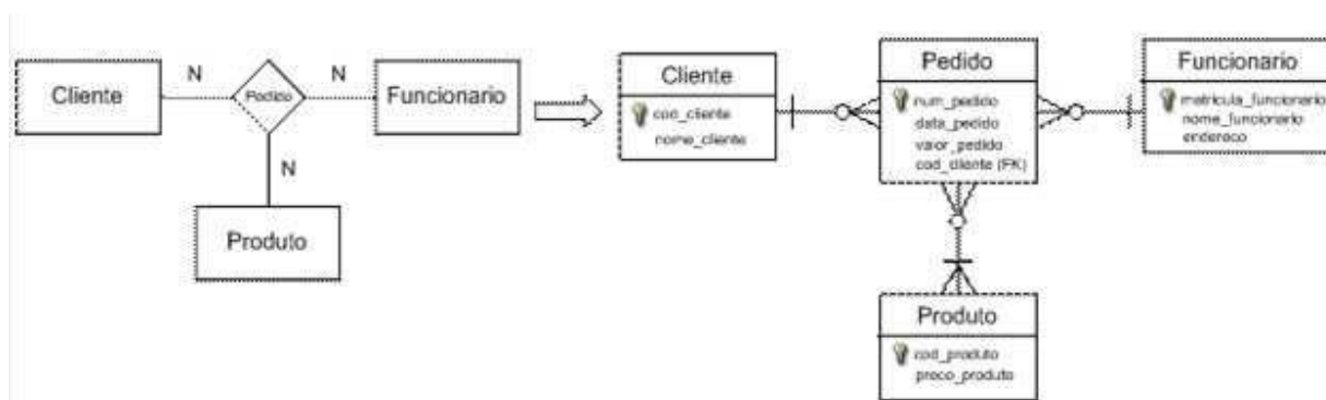
Figura 18. Mapeamento de relacionamento ternário.
