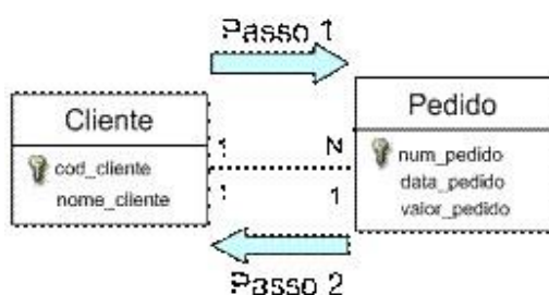
Figura 12. Entidades Cliente e Pedido – Passo 2.
