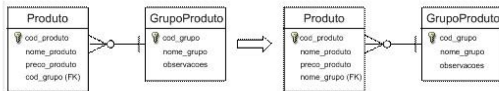
Figura 26. Exemplo de desnormalização.
