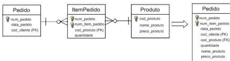
Figura 25. Tabela desnormalizada.
