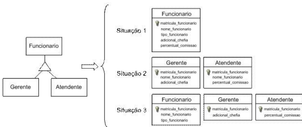
Figura 16. Generalização / Especialização.
