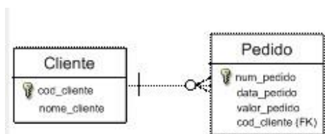
Figura 14. Entidades Cliente e Pedido – Final.
